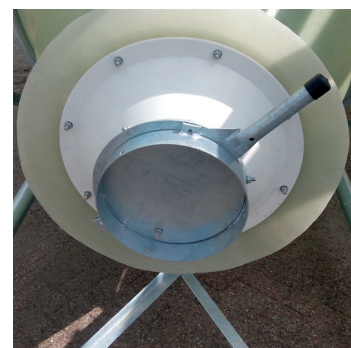
Aftapschuif
